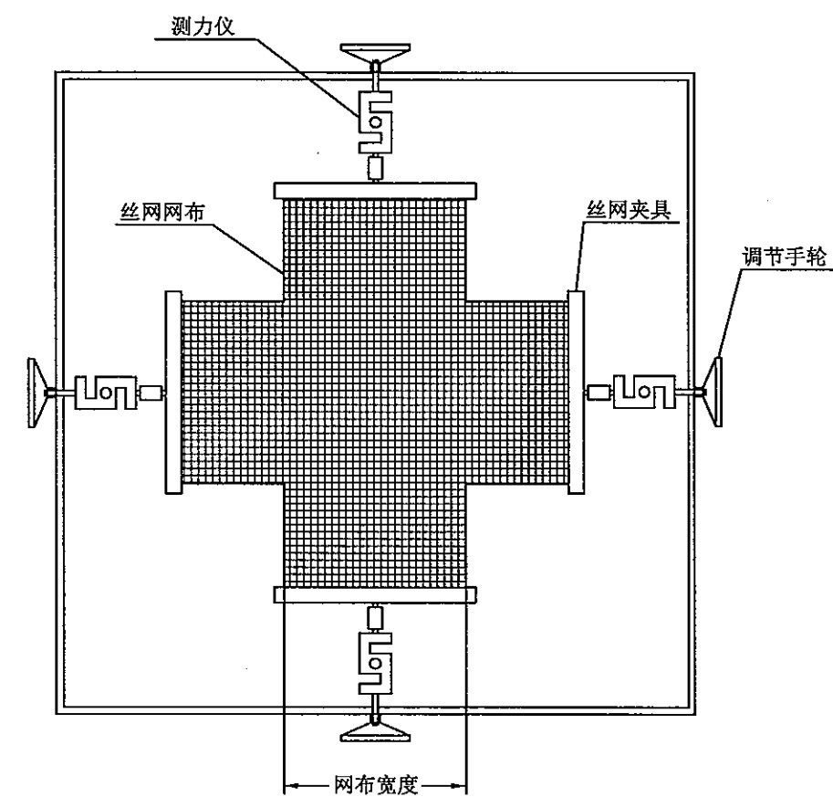
图 D.1 一种典型的丝网张力标准装置示意图
